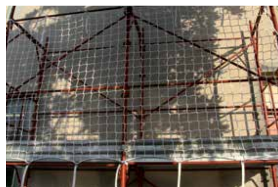
Art. 00316 - Ancorante con gancio a ricciolo per reti anticalcinacci tassello in acciaio foro \varnothing 12mm filetto 9mm
