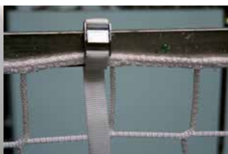
00320 tiranti/blizz altezza mm 25, lunghezza cm.50, nastro poliestere ht bianco, con fibbia in acciaio,carico di rottura minimo 800 kg
