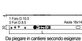
394 zincato L=755
