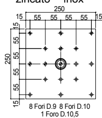
391 zincato
