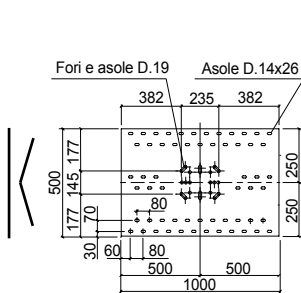
405R piana
