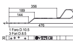
397 zincato
