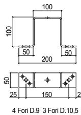
392 zincato
