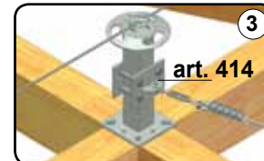
Modalità di fissaggio per ridurre i momenti flettenti sulla struttura di supporto
