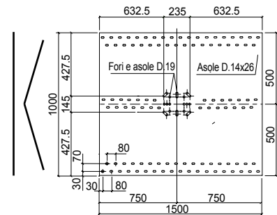
405V piana
