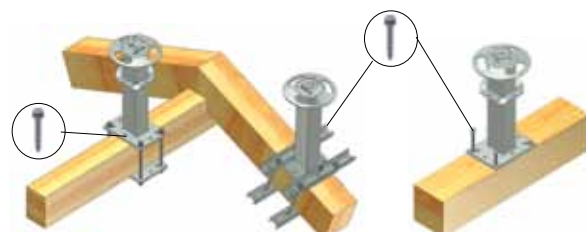
Staffaggio con barre filettate, contropiastre o profili di riscontro (vedi NOTA )
