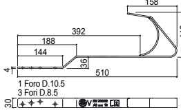
398 zincato
