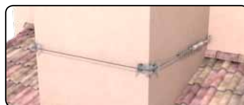
Caso di linea vita a parete su 3 lati: ancoraggi 601-601C come estremità e 601H-601L come intermedio.
